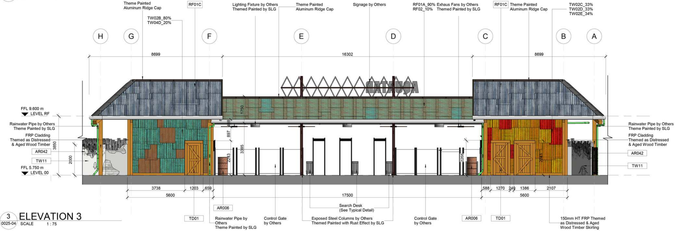
2 ELEVATION 2 0025-04 SCALE 1:75
